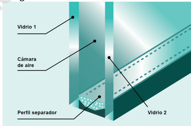
Imagen N° 27: Sistema doble vidriado hermético.
