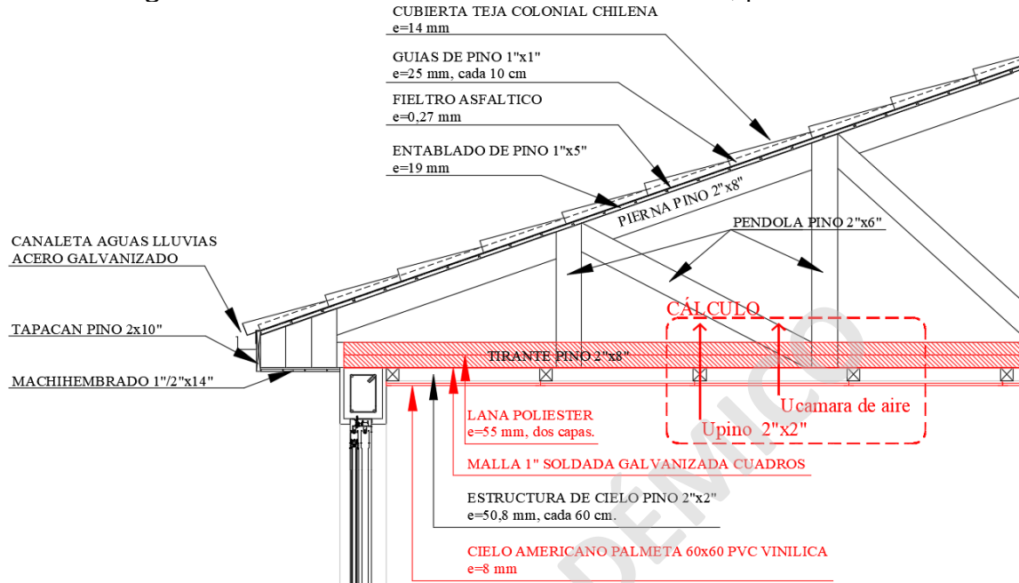
Imagen N° 65: Solución de acondicionamiento térmico, para techumbre.
