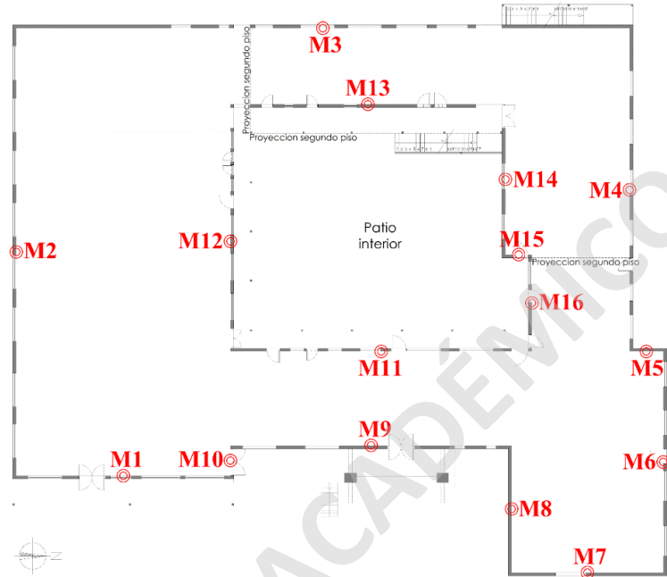
Imagen N° 57: Planta primer piso, identificación de muros perimetrales.
