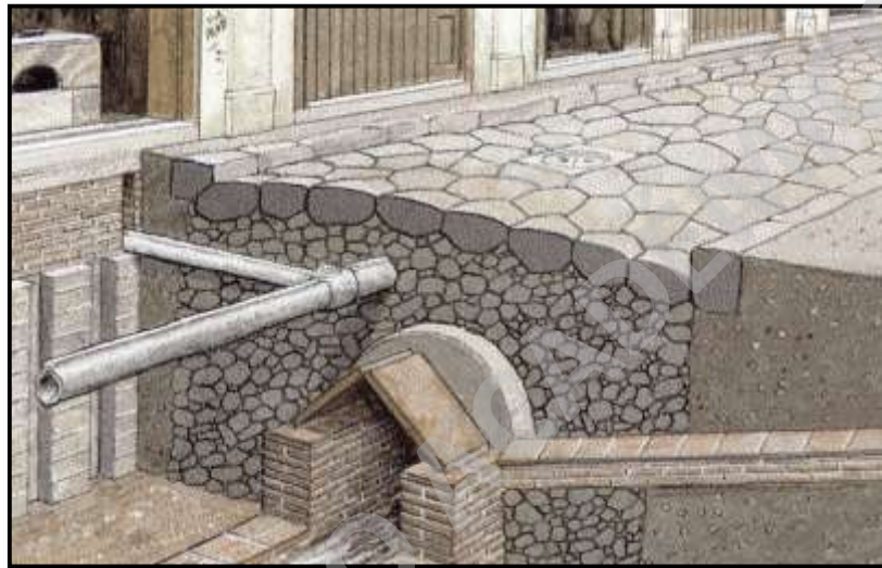
Imagen N° 9: Diseño de Alcantarillado Romano
