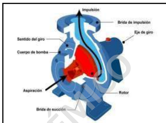
Imagen N° 29: Bomba Centrífuga
