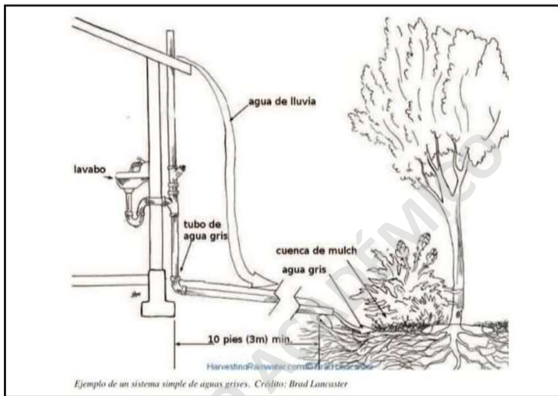
Imagen N° 32: Sistema Simple de Aguas Grises
