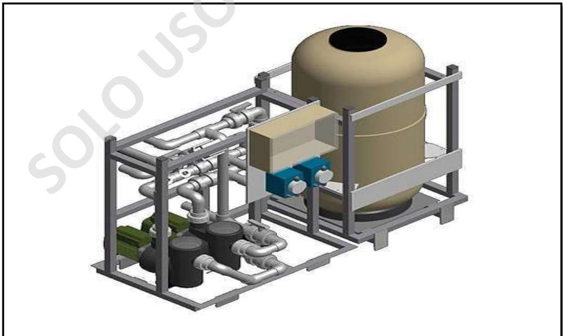
Imagen N° 42: Sistema Ecostep Pro
