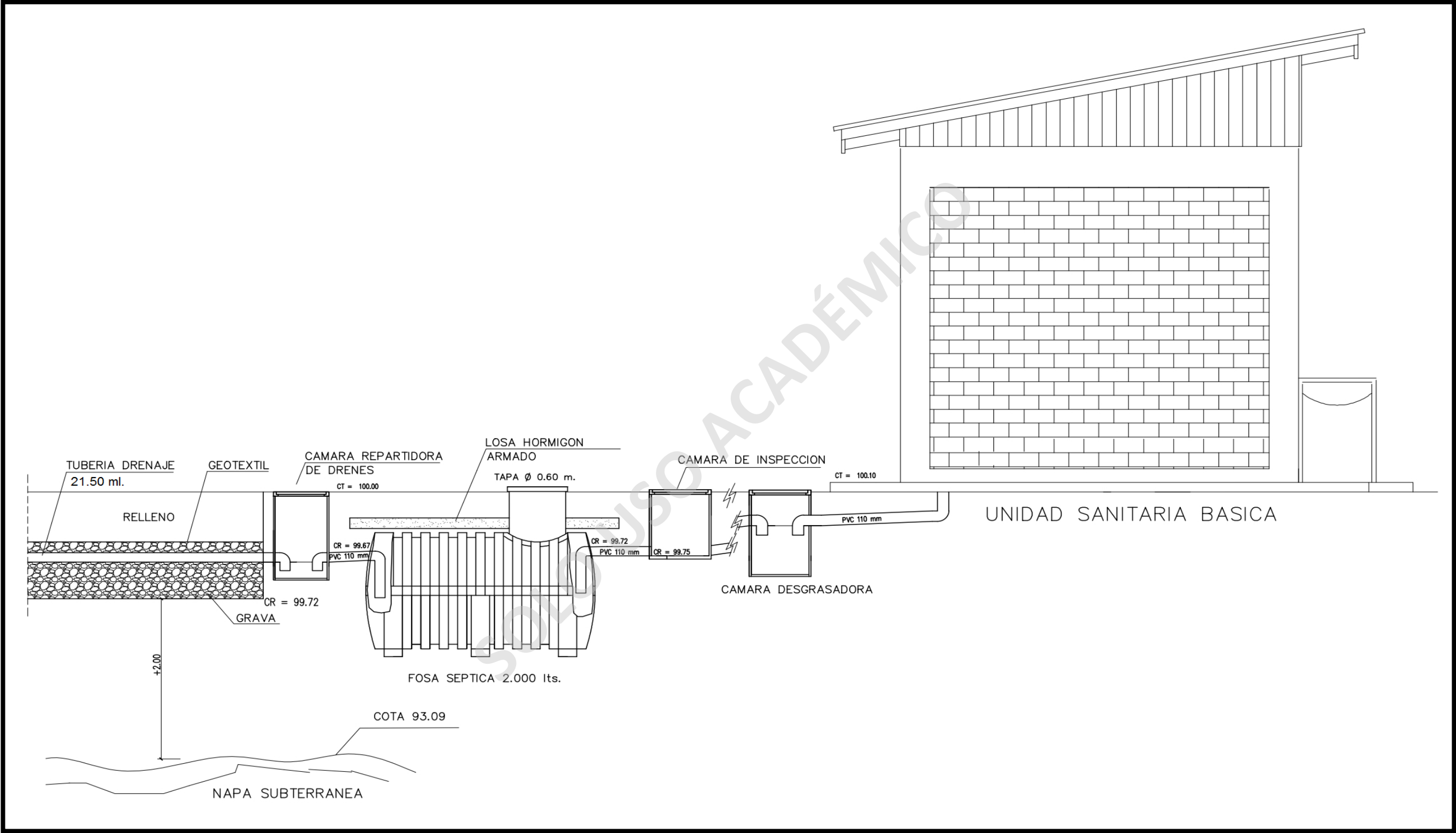
ANEXO N° 6.- Unidad sanitaria básica con sistema fosa - dren, con requisitos de instalación a profundidad.
