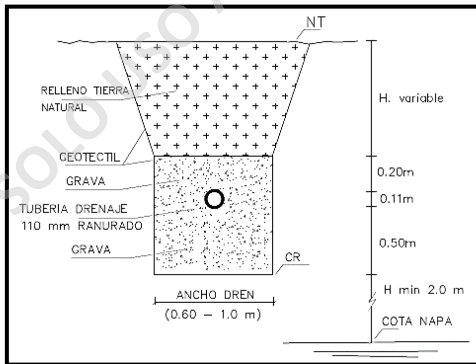
Imagen N° 16: Corte Dren de infiltración.
