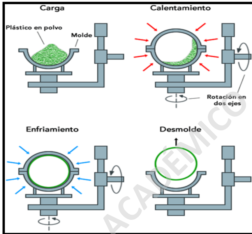
Imagen N° 5: Proceso de Rotomoldeado.
