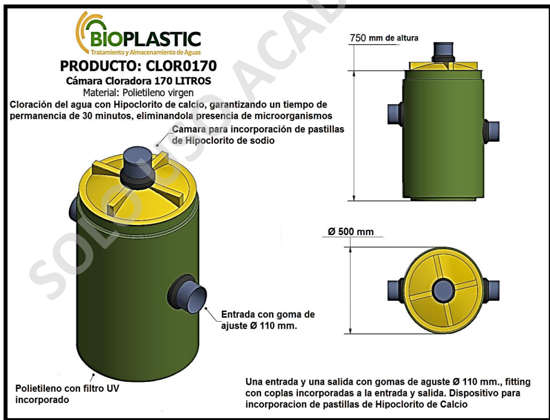
Imagen N° 18: Cámara Cloradora.
