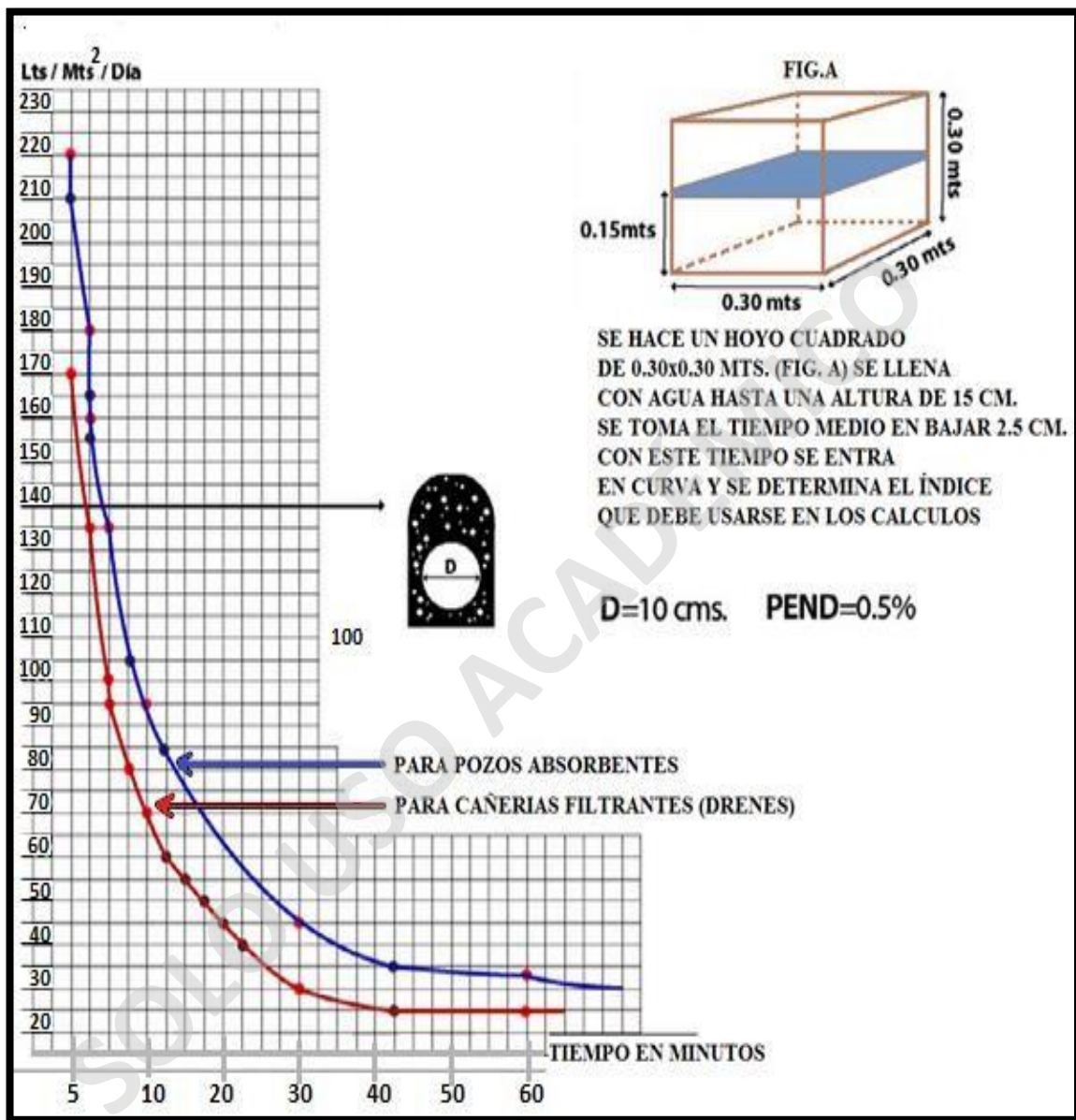
Imagen N° 12: Ensaye para determinar índice de absorción de pozos absorbentes y drenes de infiltración.
