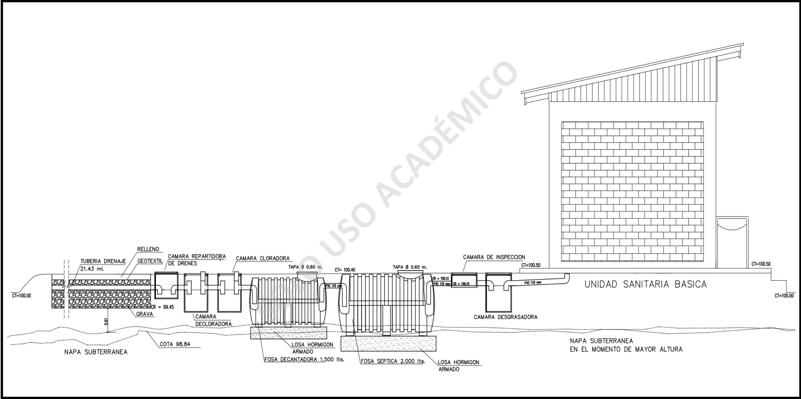
ANEXO N° 8.- Unidad sanitaria básica con sistema fosa - dren, con presencia de napa freática de 1.0 a 2.0 m., respecto el nivel de terreno
