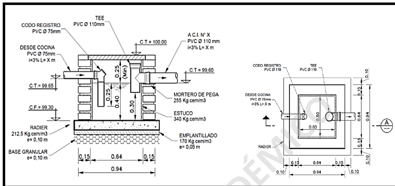
Imagen N° 2: Cámara Interceptora de Grasa y Jabones de Albañilería.
