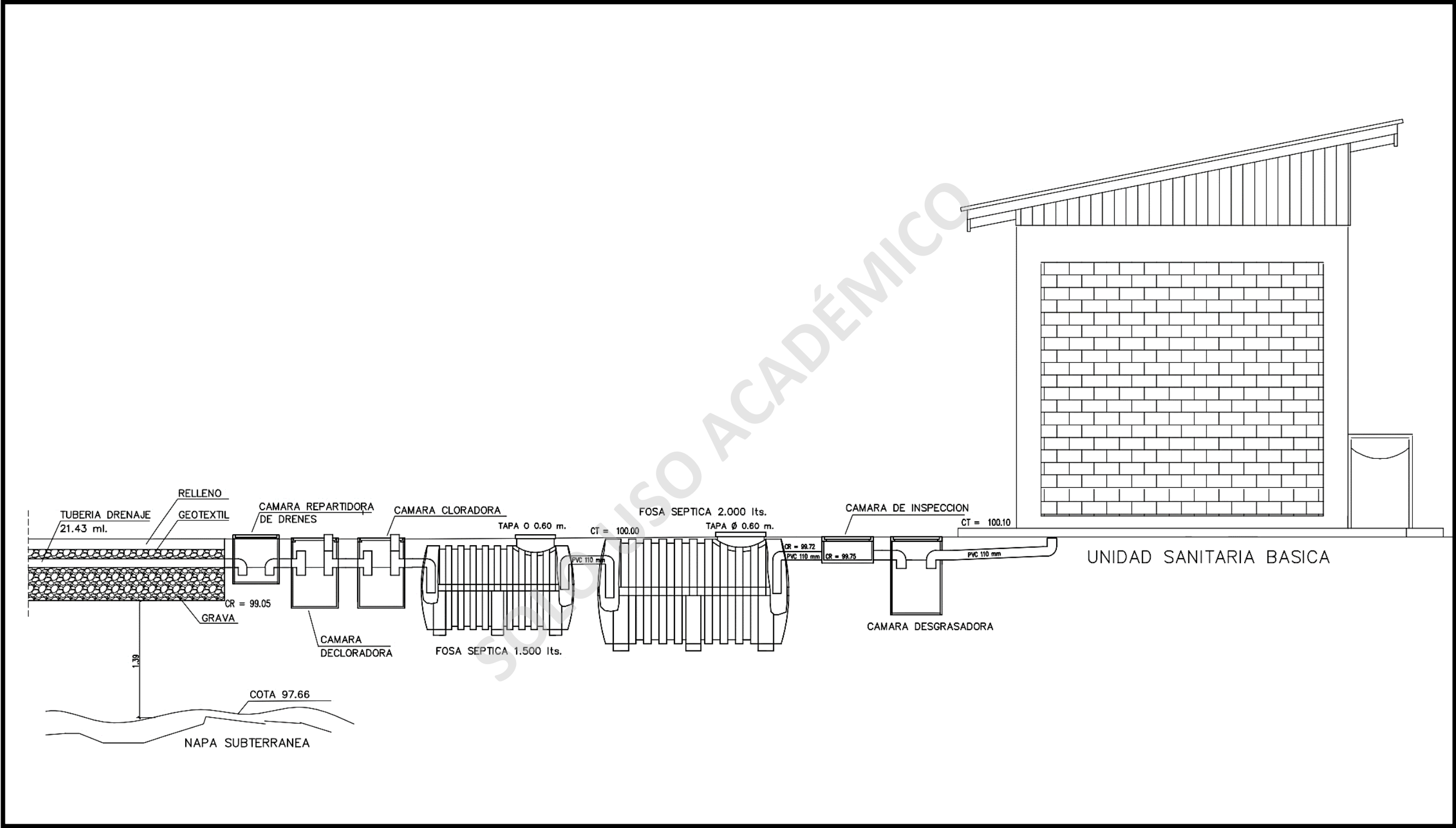
ANEXO N° 7. -Unidad sanitaria básica con sistema fosa - dren, con presencia de napa freática a menos de 2.0 m., respecto de la base del dren.
