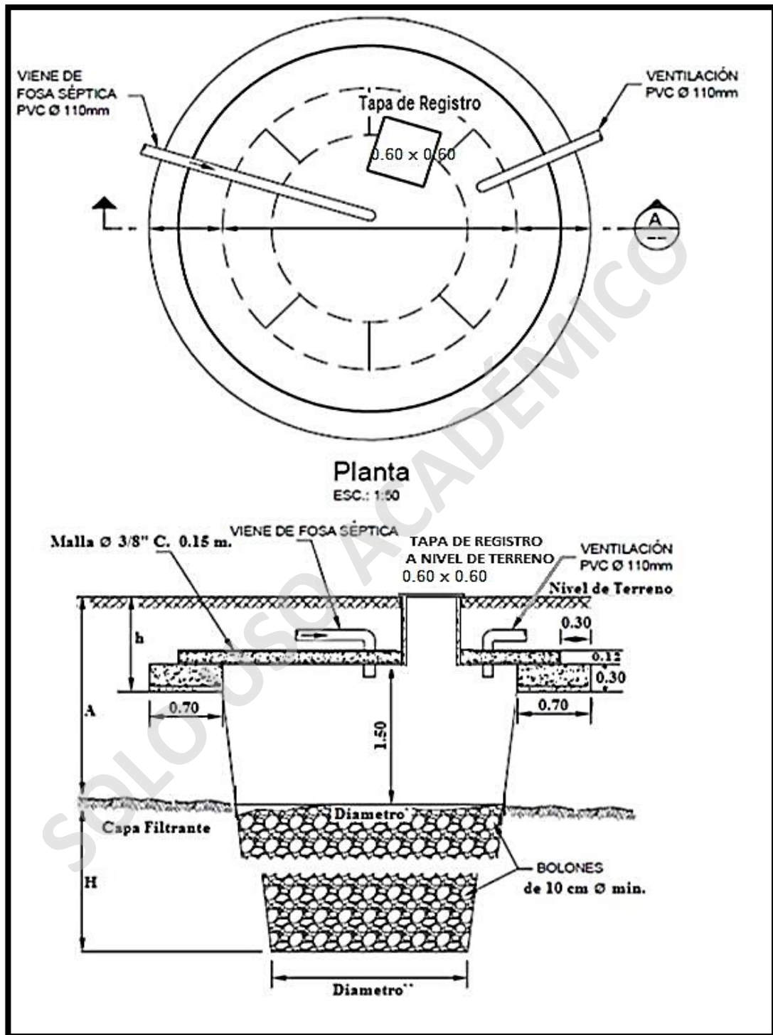
Imagen N° 13: Pozo Absorbente.
