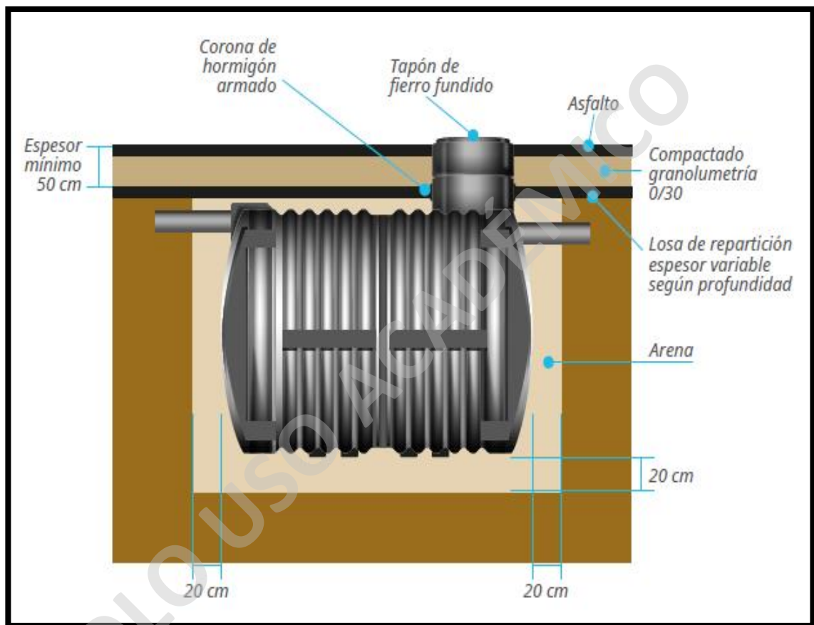
Imagen N° 9: Fosa Séptica Instalada bajo zona de circulación vehicular.
