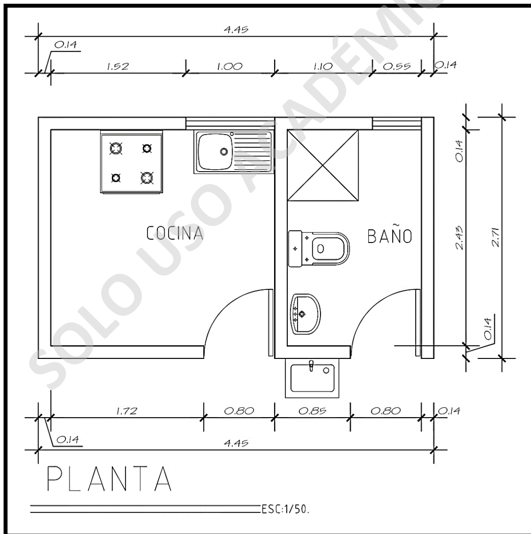
Imagen N° 21: Planta Unidad Sanitaria Básica.
