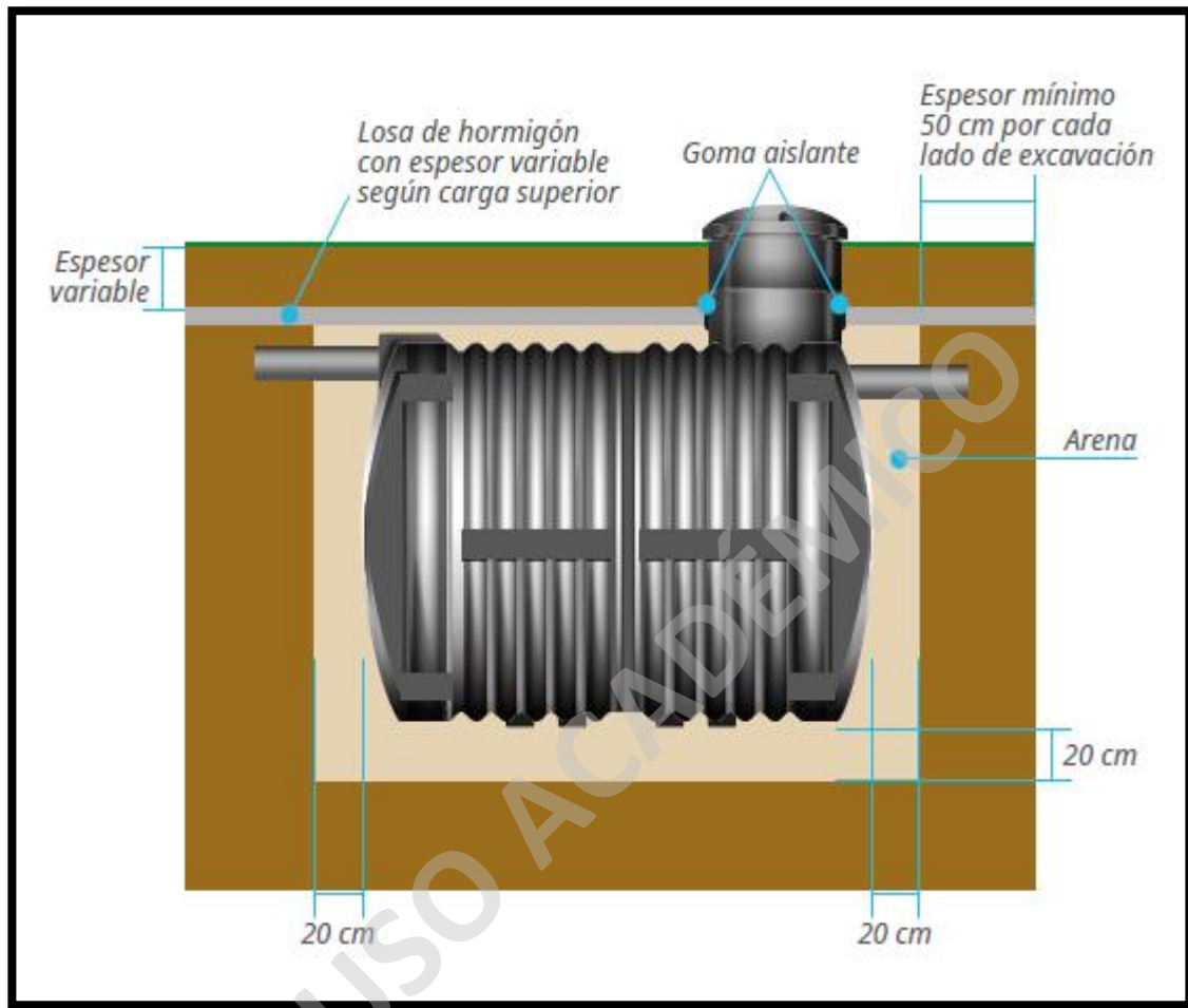
Imagen N° 8: Fosa Séptica Instalada a más de 0.3 m., respecto del nivel de terreno.
