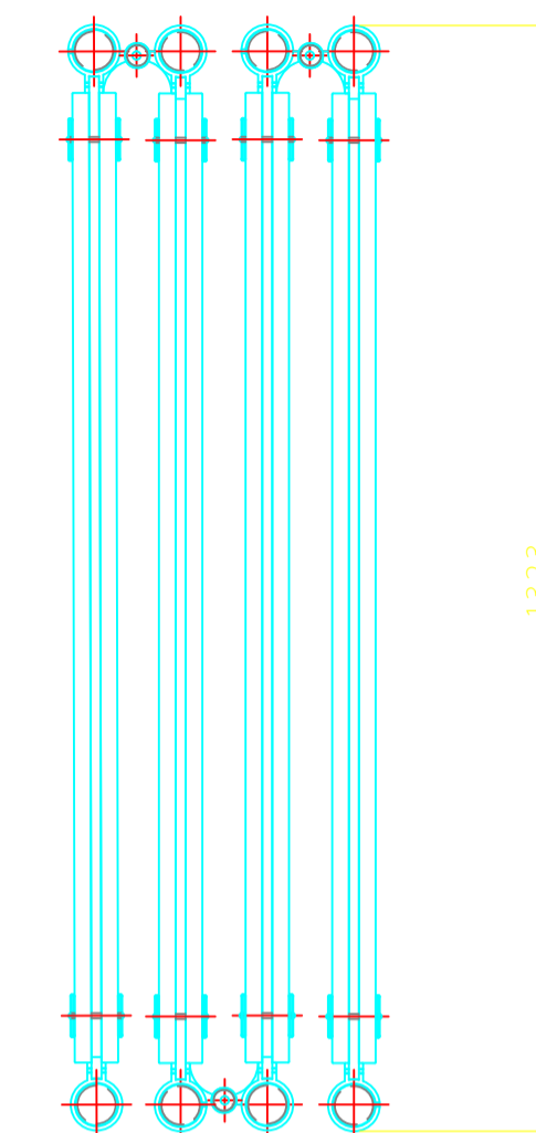
Vista Superior Plegada
