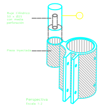
Perspectiva Escala 1:2
