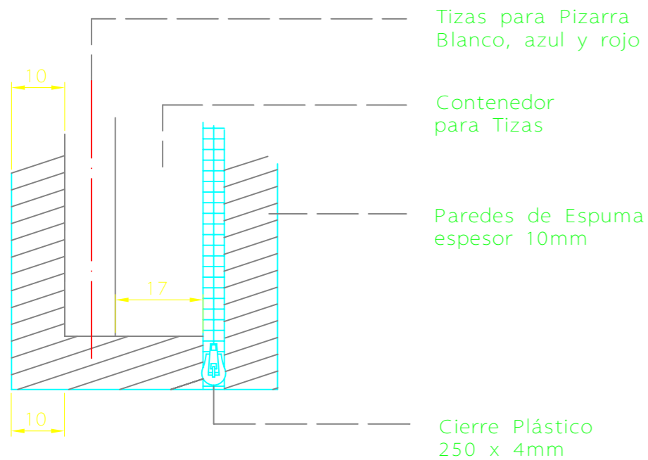
Detalle 2 Esc. 1:1
