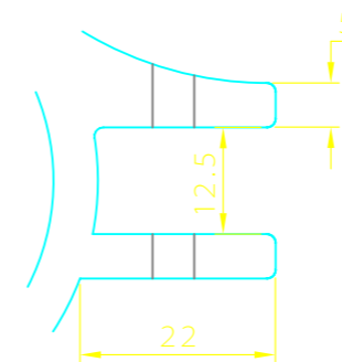
Detalle 2 Esc. 1:1
