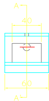
Vista Superior
