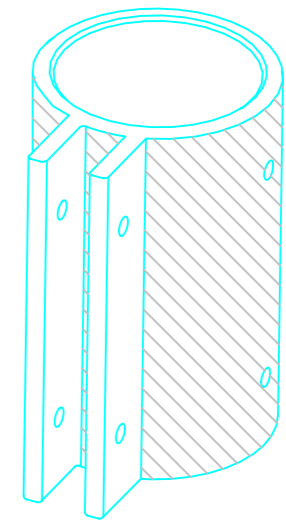
Perspectiva Escala 1:2
