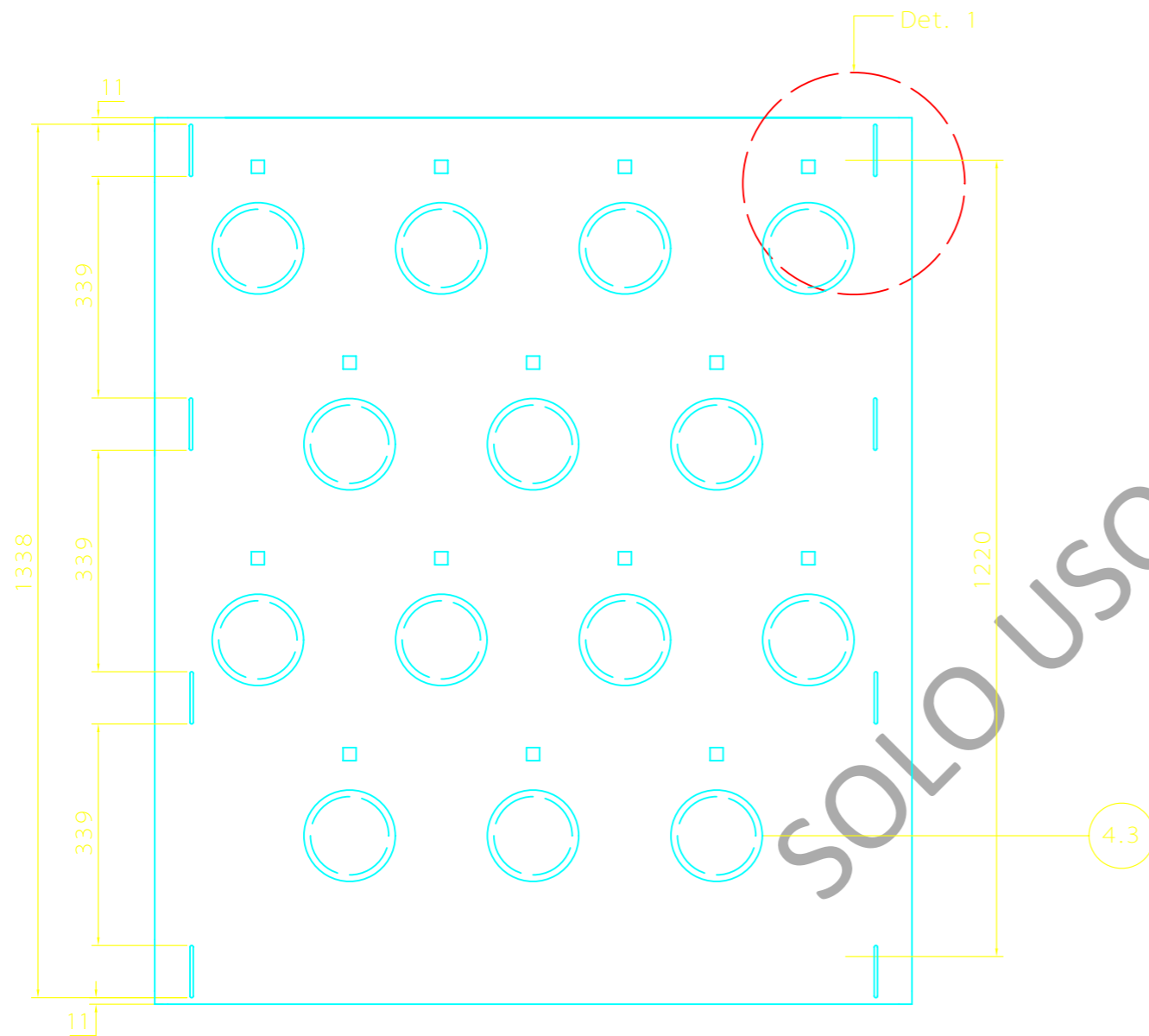
Vista Superior
