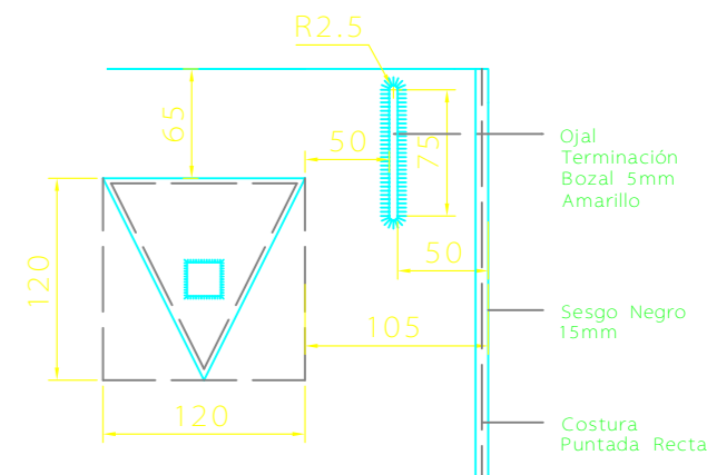
Detalle 2 Esc. 1:5
