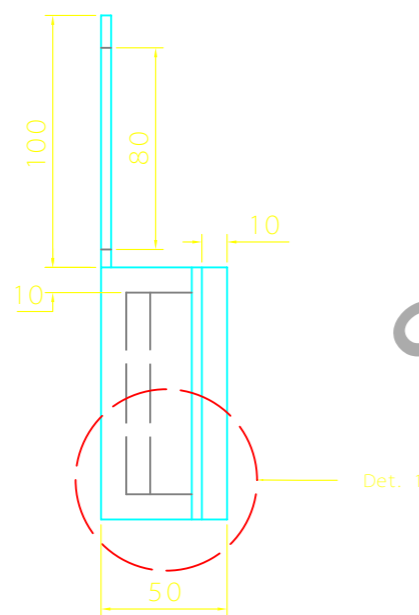
Vista Lateral Izquierda
