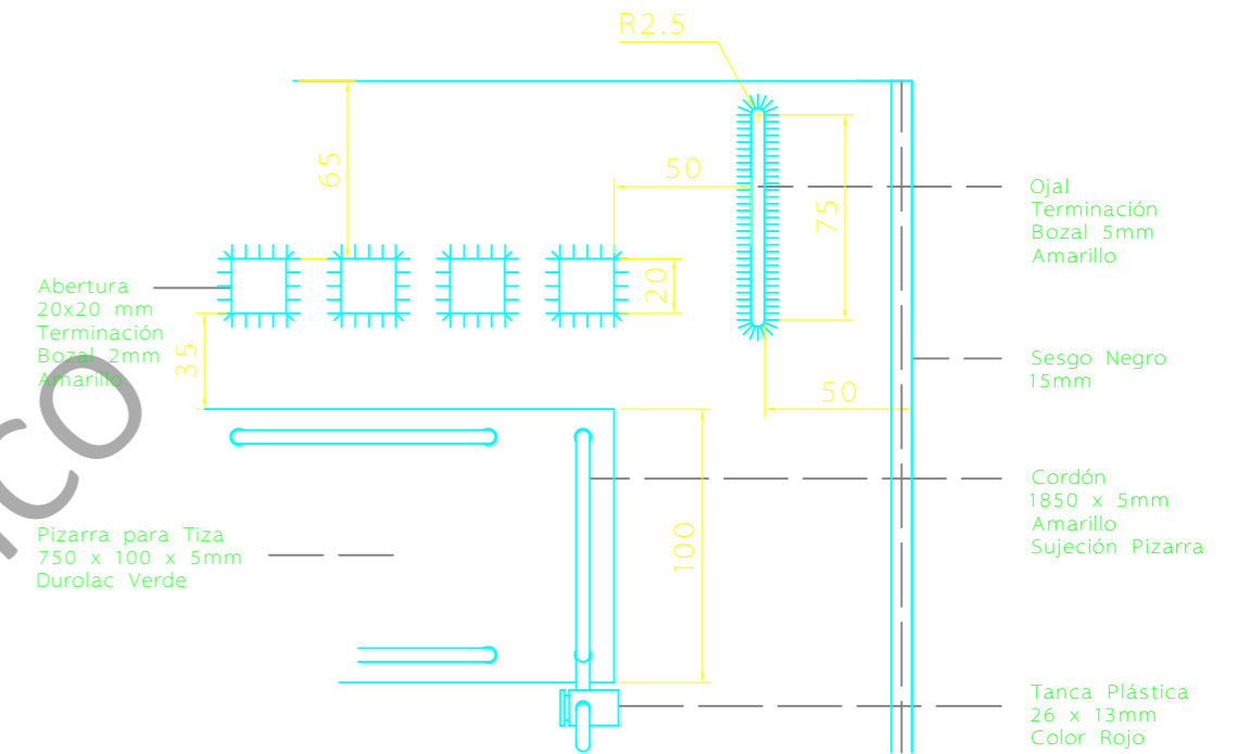
Detalle 1 Esc. 1:3
