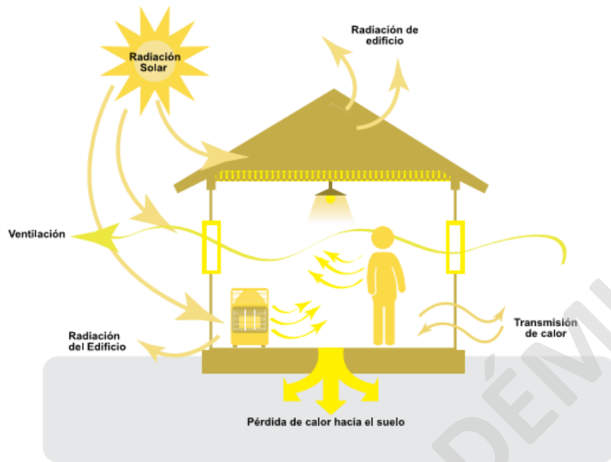
Imagen N° 8: Procesos de transferencia de calor en una vivienda.
