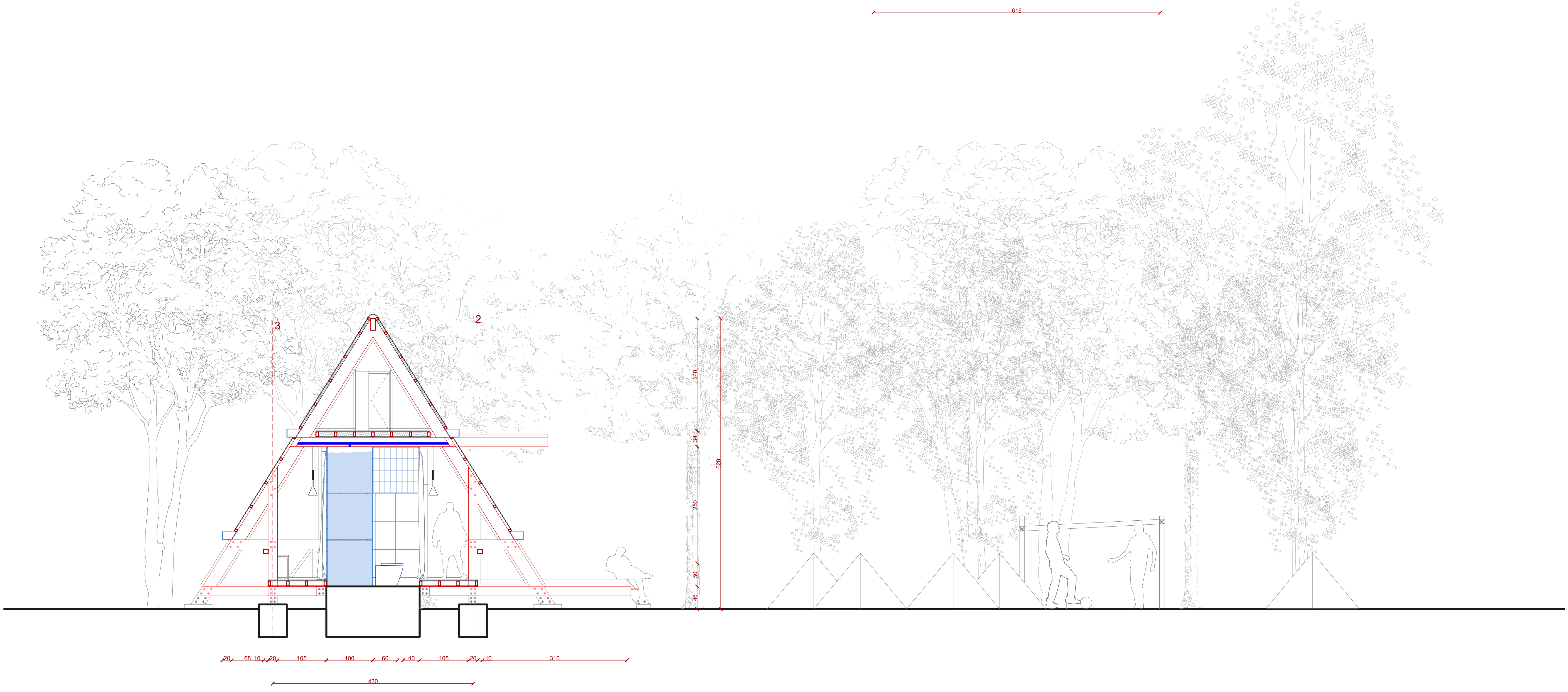
Corte D_D' - esc 1/50
