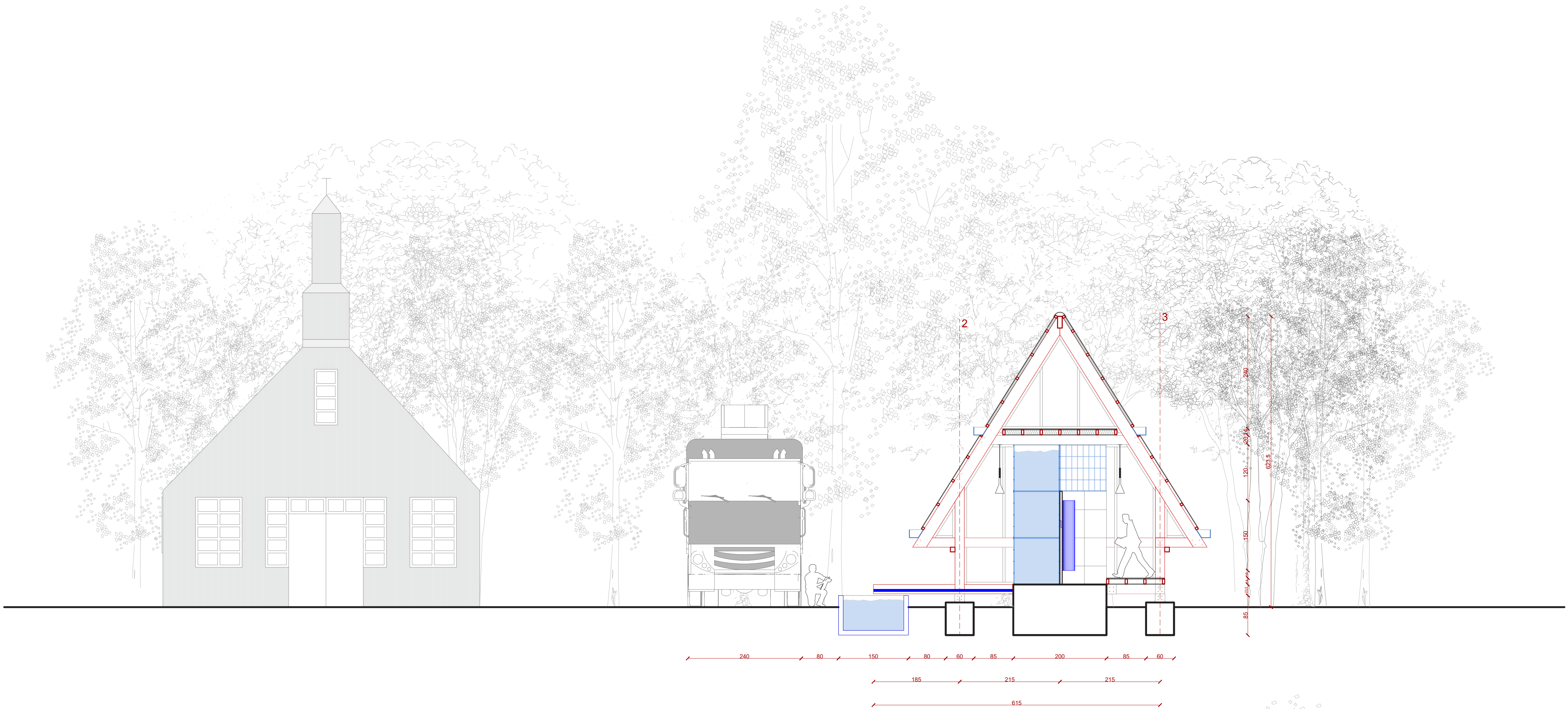
Corte C_C' - esc 1/50
