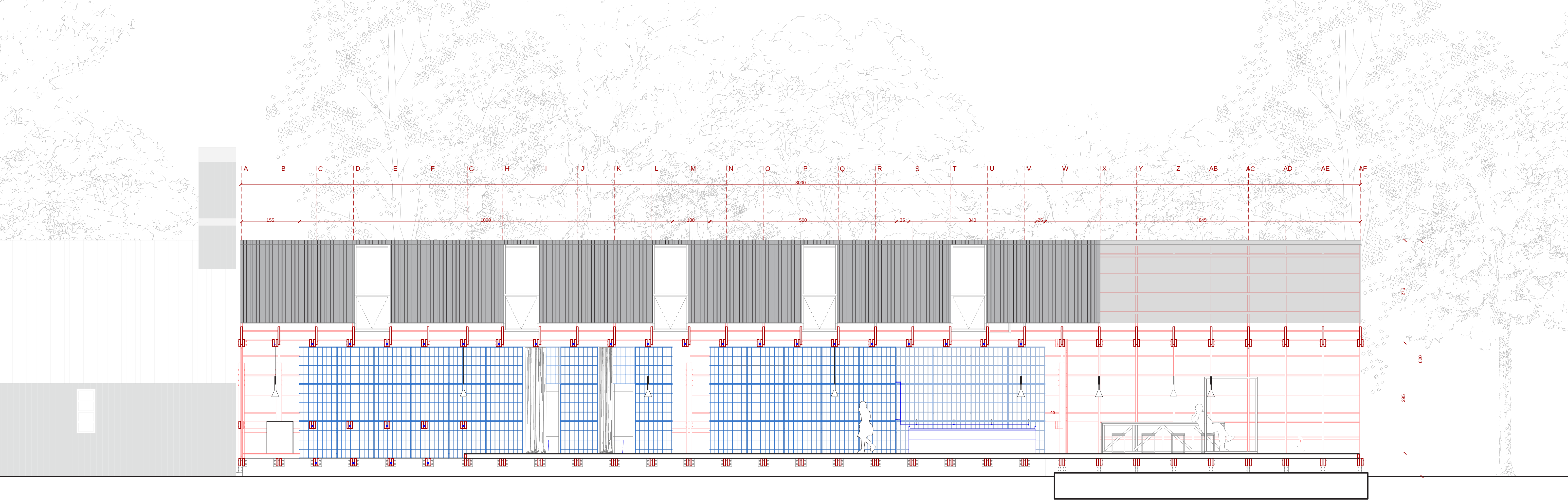
Corte G_G' - esc 1/50
