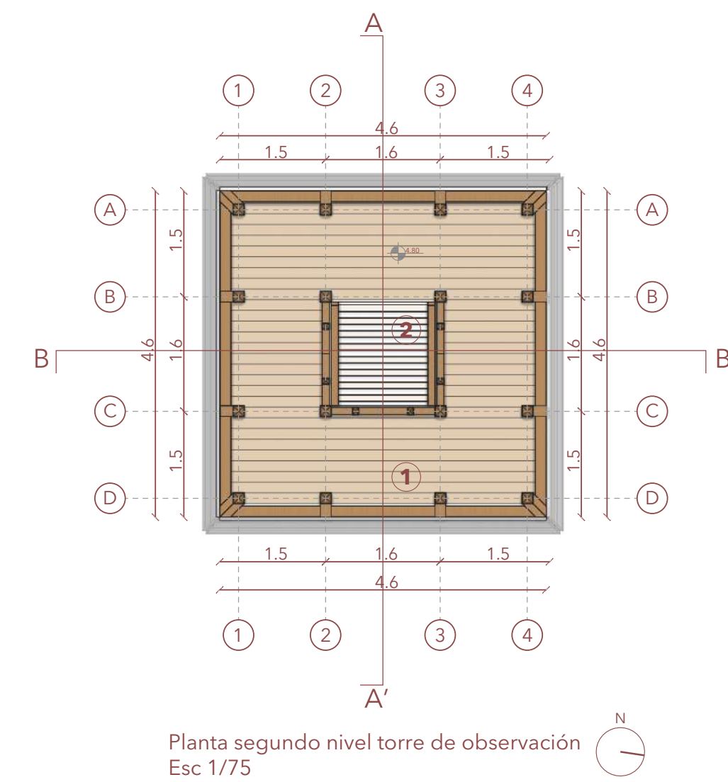
Planta segundo nivel torre de observación Esc 1/75
