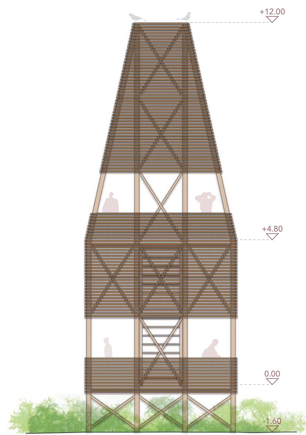
Elevación sur Esc 1/75
