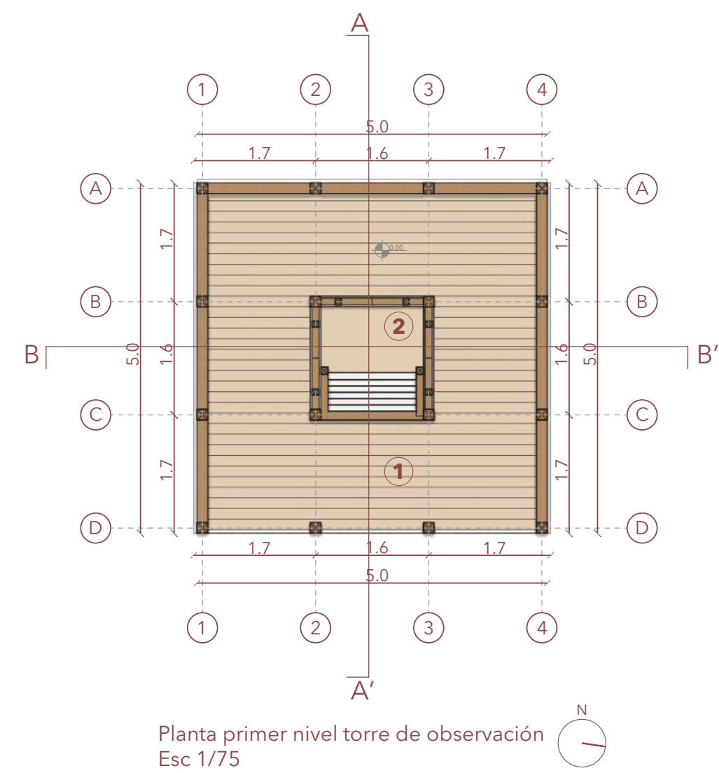
Planta primer nivel torre de observación Esc 1/75
