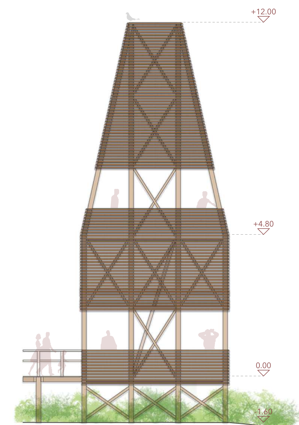
Elevación norte Esc 1/75
