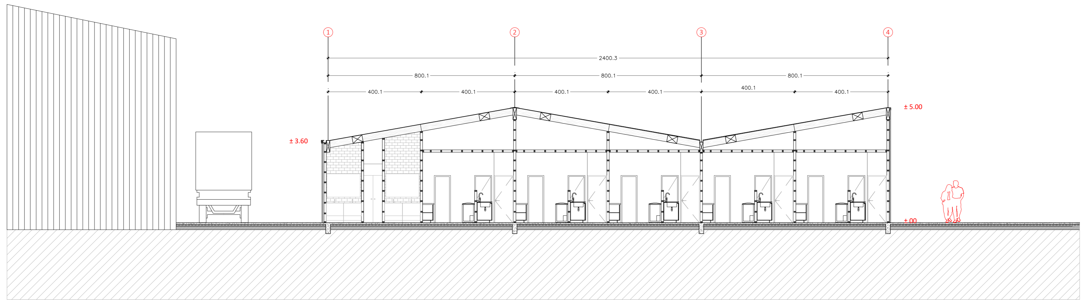
CORTE A-A
