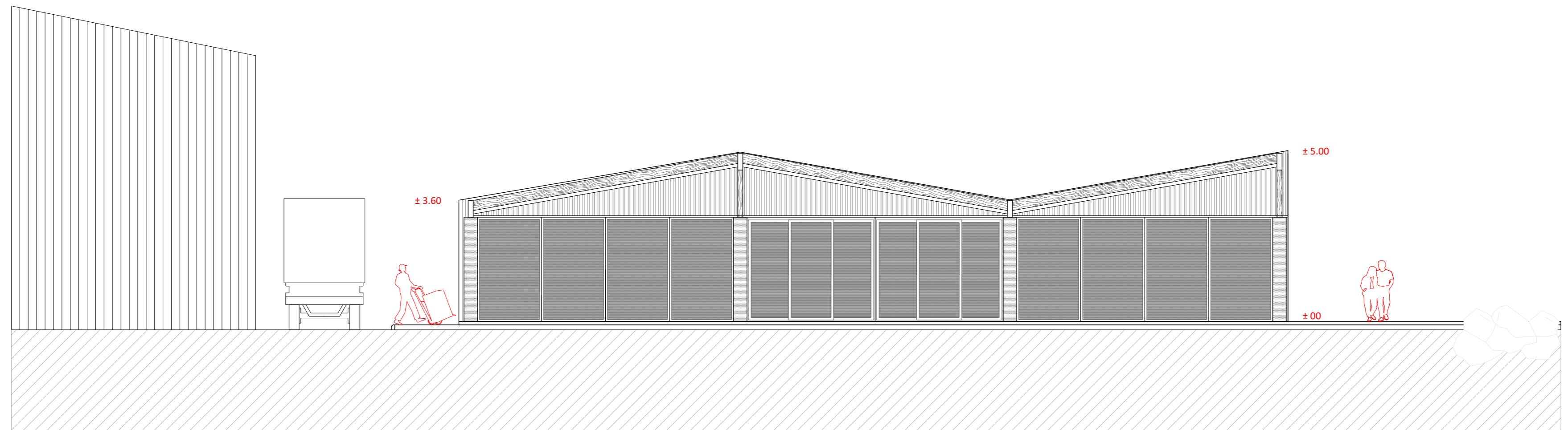
Elevación Sur
