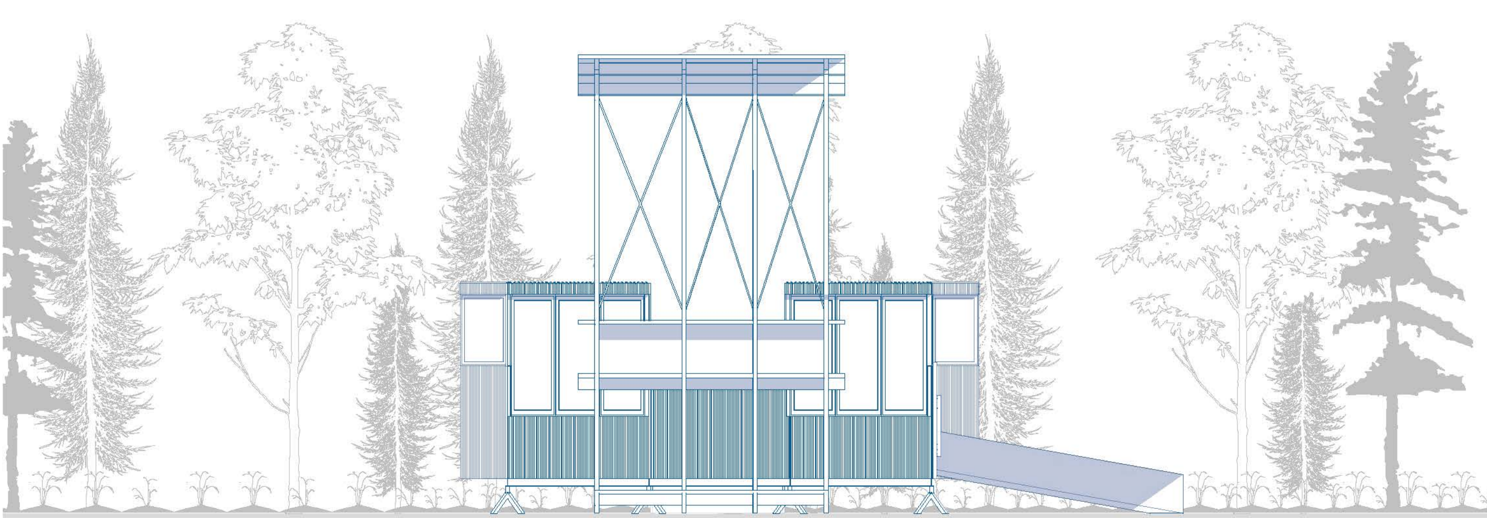
ELEVACION TRASERA
