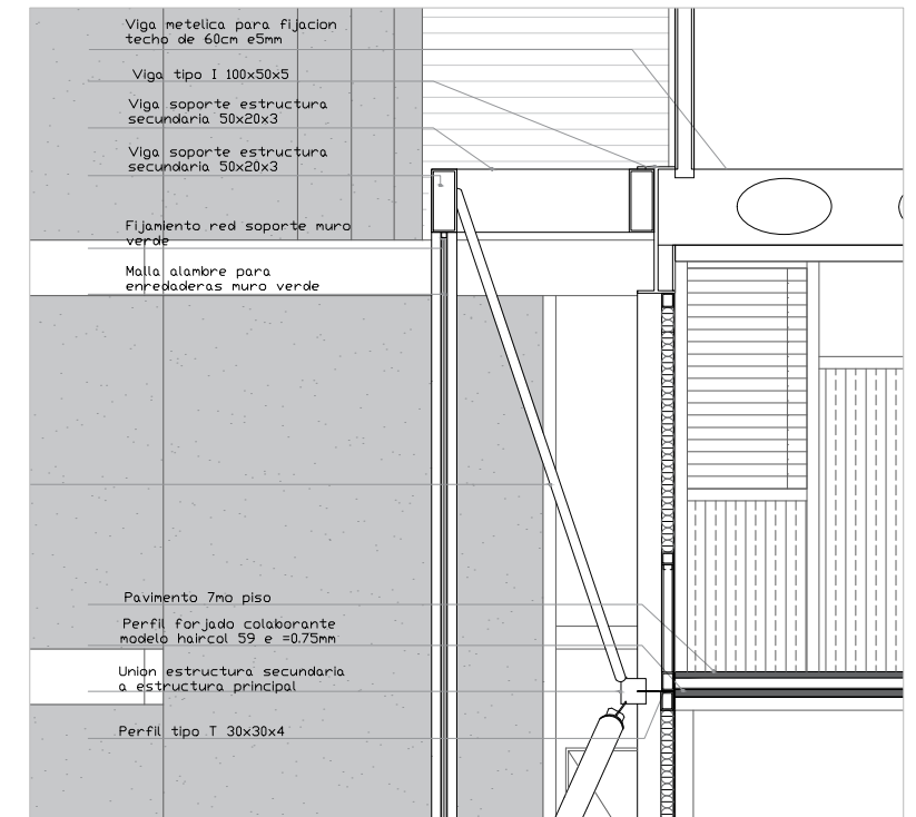
DETALLE 3
