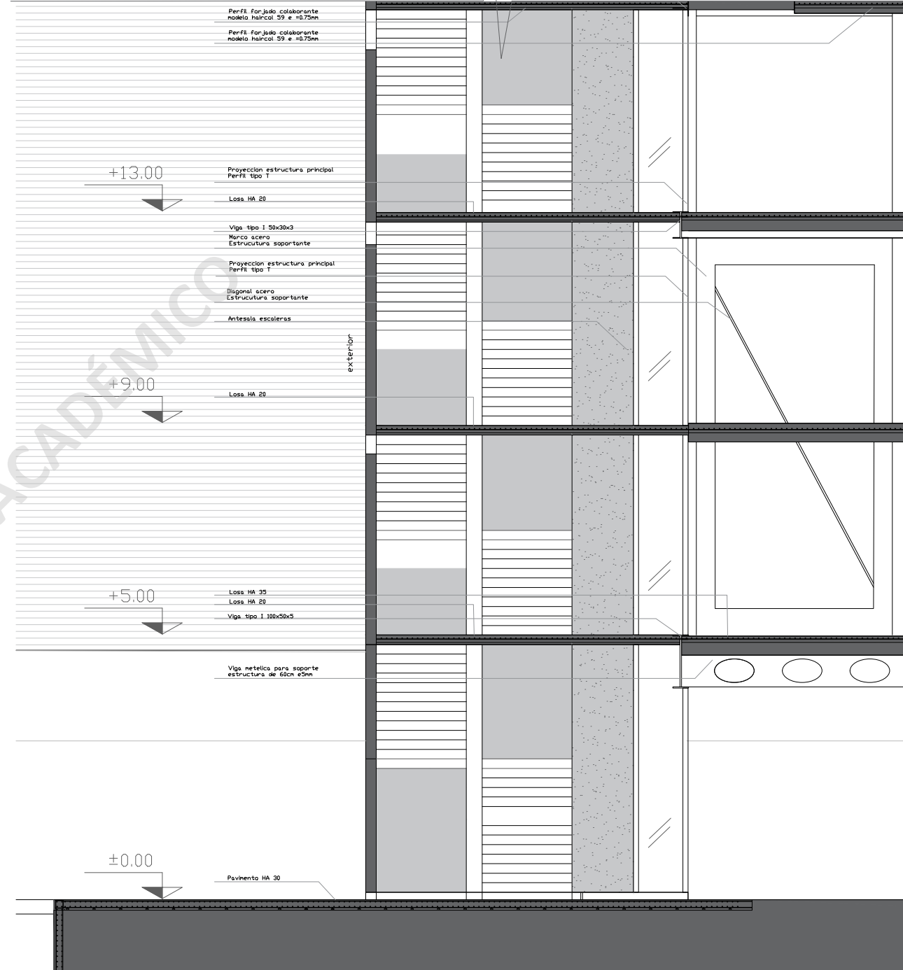
CORTE ESCANTILLON 3
