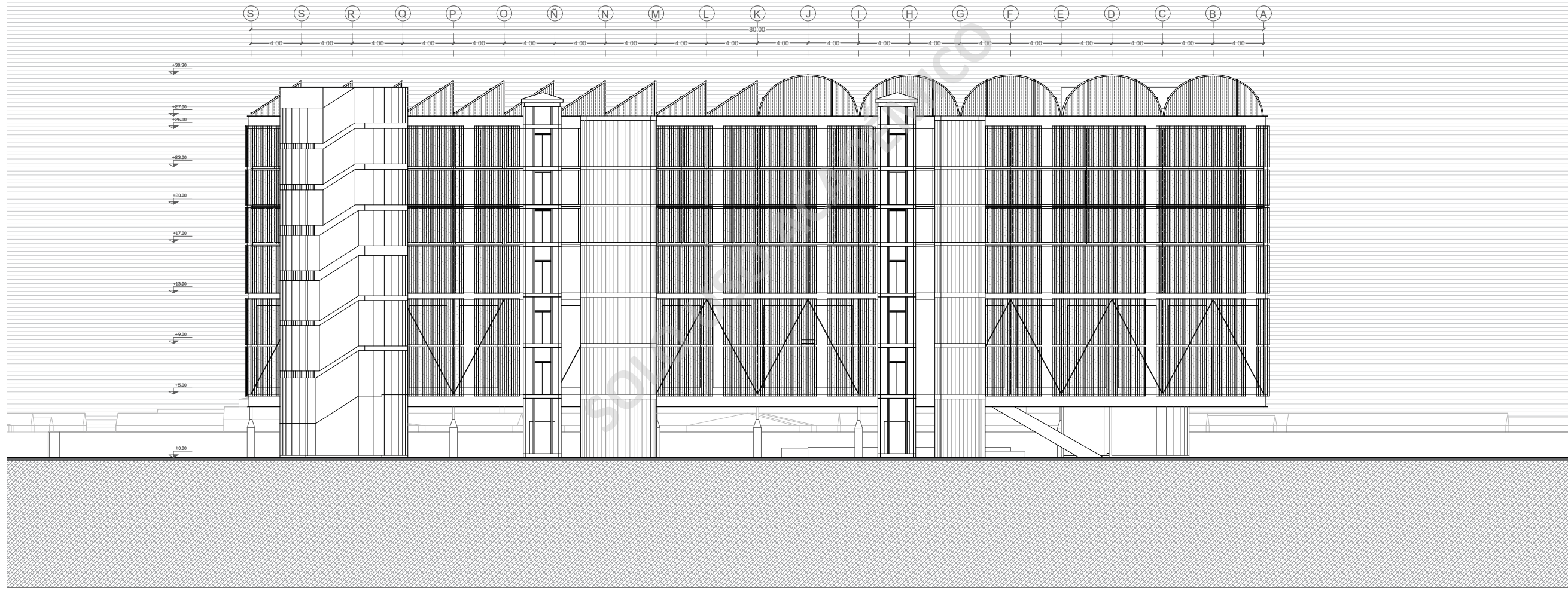
ELEVACION ORIENTE
