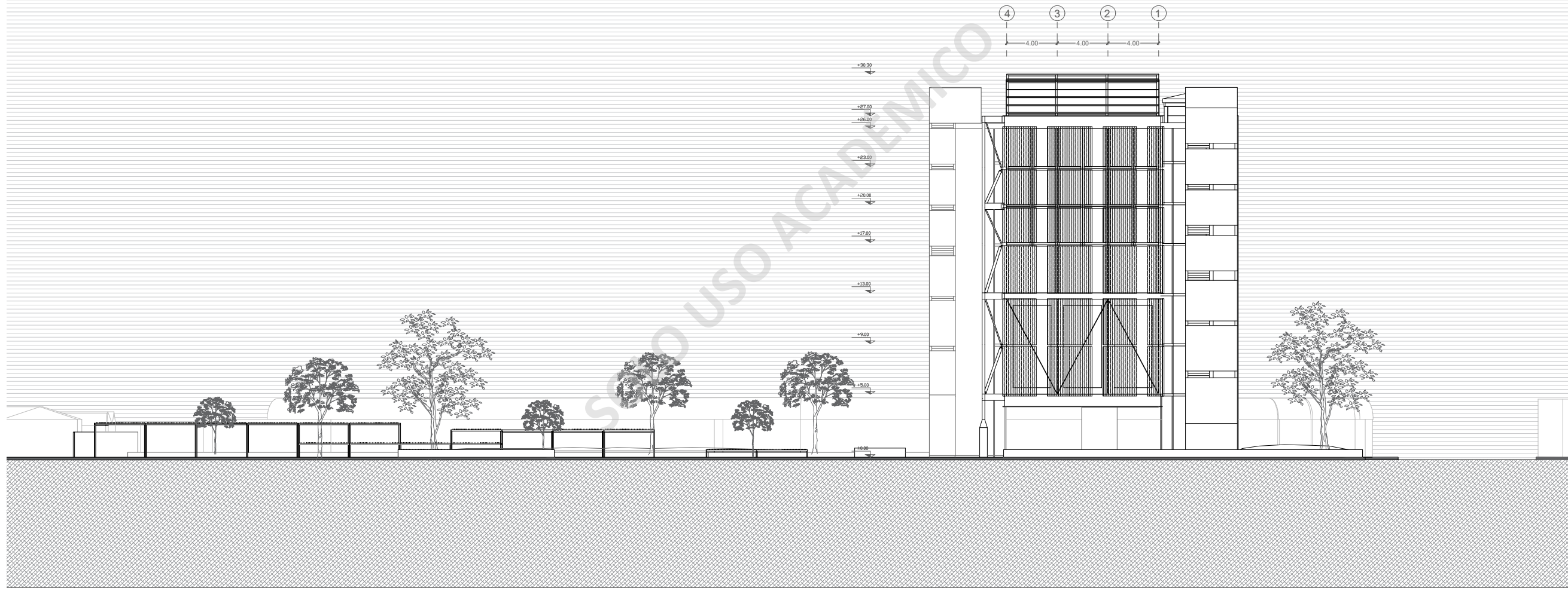
ELEVACION SUR
