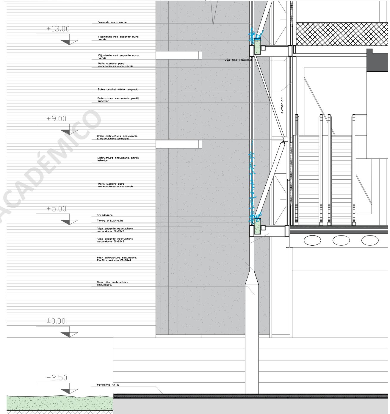
CORTE ESCANTILLON 2
