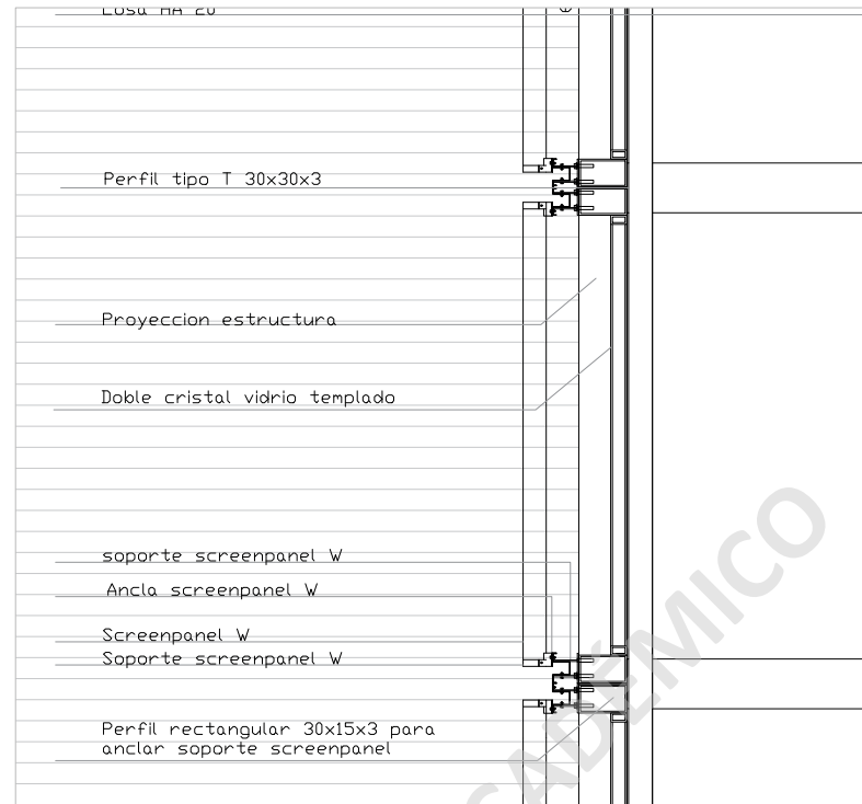
DETALLE 2
