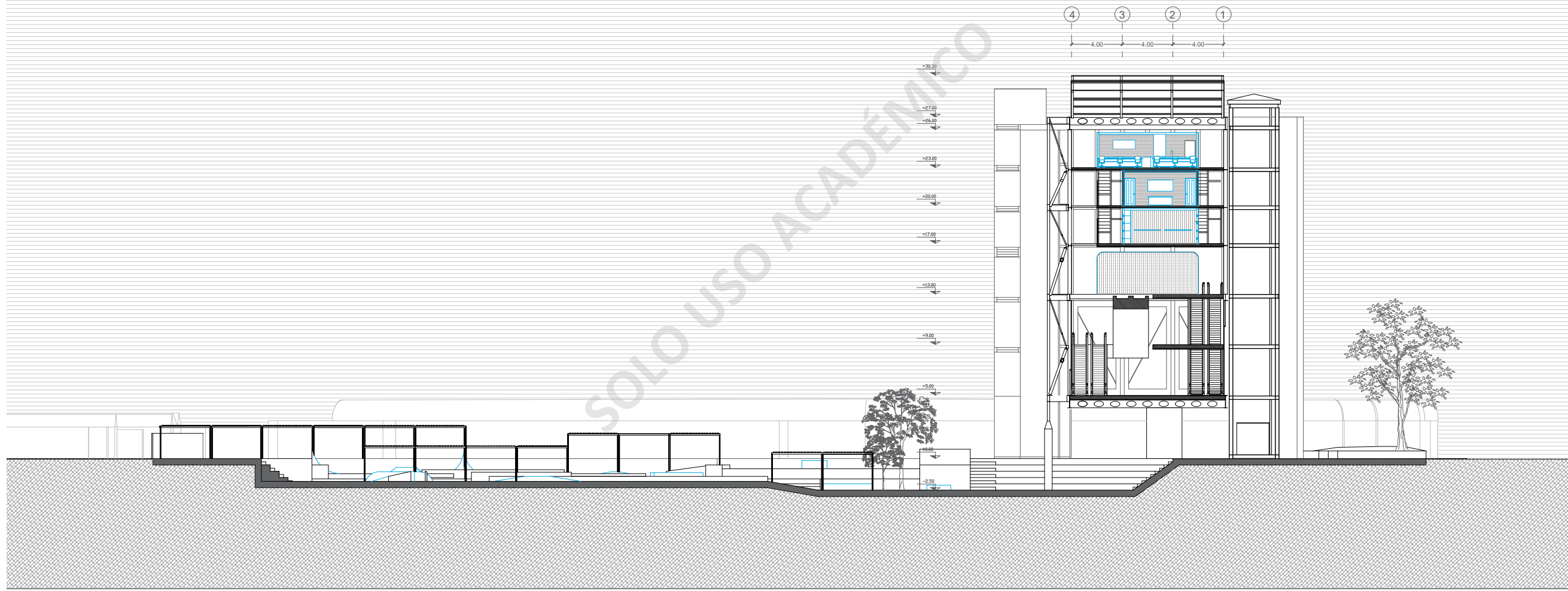
CORTE B-B
