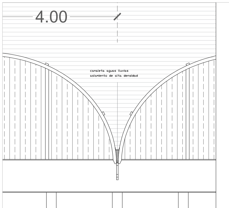
DETALLE 4
