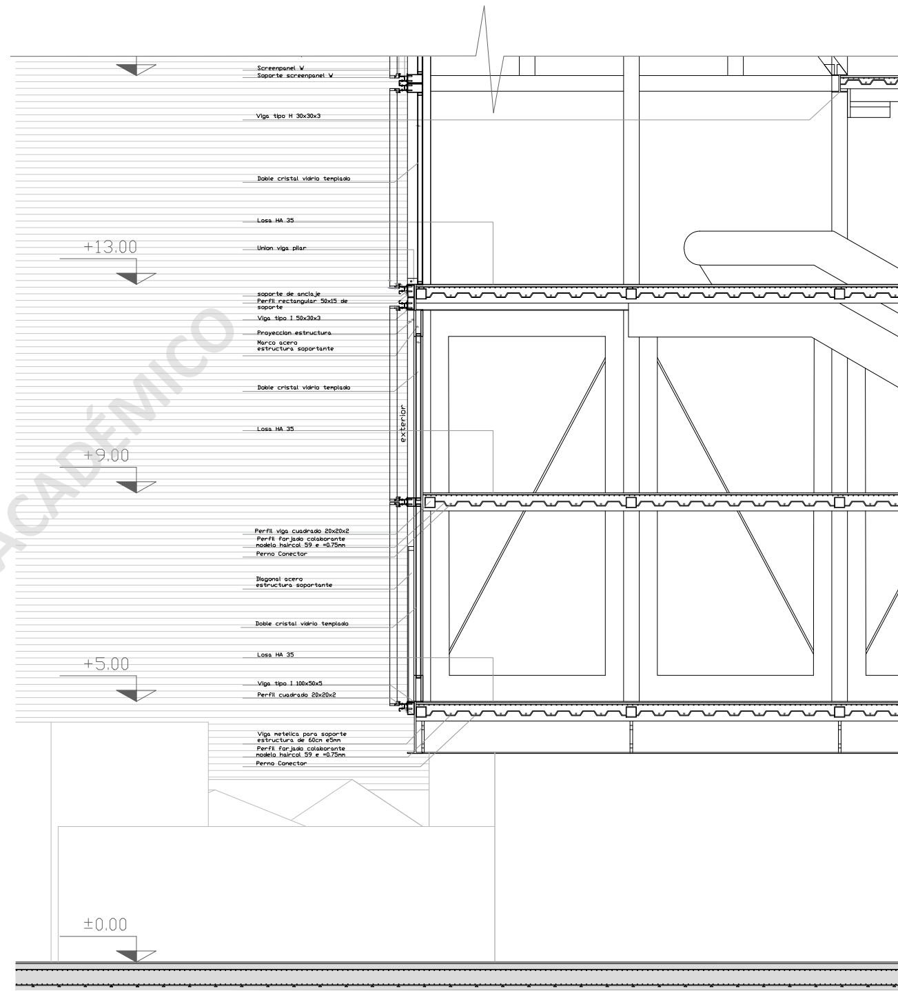
CORTE ESCANTILLON 1
