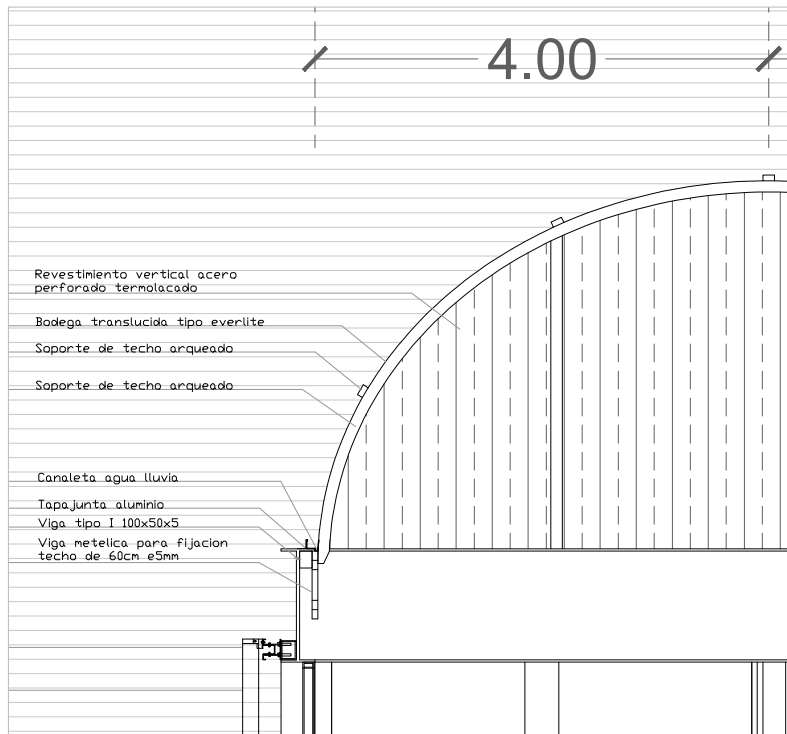
DETALLE 1
