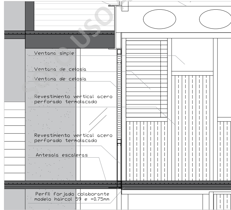
DETALLE 5
