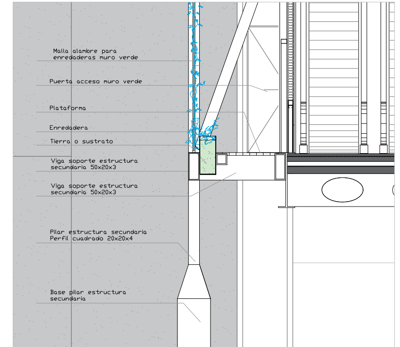
DETALLE 6
